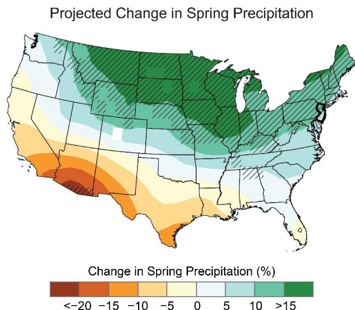
Fig. 25: Cambio previsto en las precipitaciones de primavera 66
